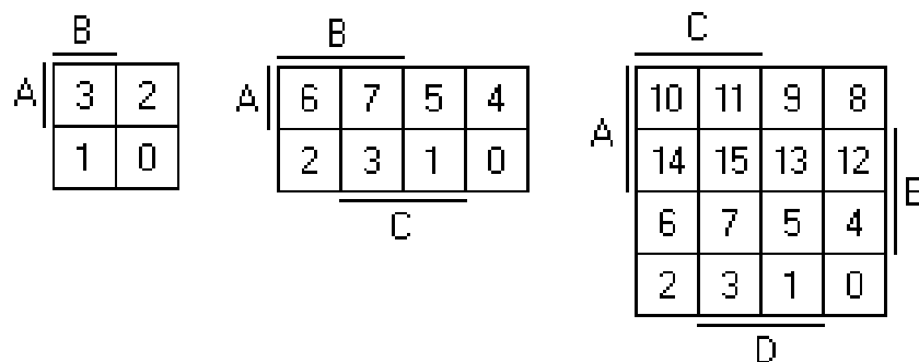
Рис. 4.1. Нумерація таблиць Карно для 2, 3 і 4 змінних
