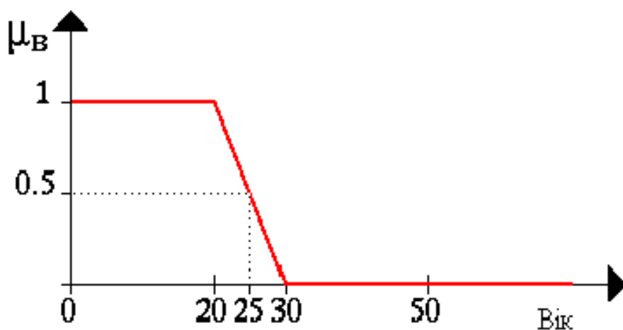
Рис. 2.2. Характеристична функція множини молодих людей
