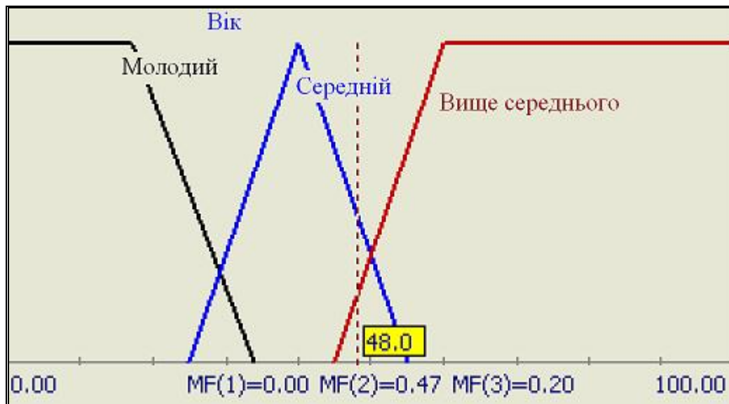
Рис. 2.8. Опис лінгвістичної змінної «Вік».
