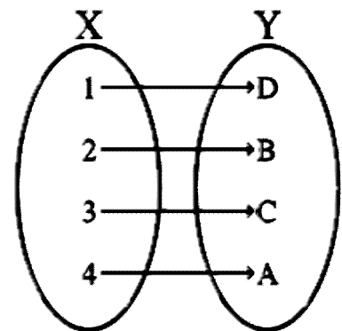
Рис. 1.2. Бієктивна функція
