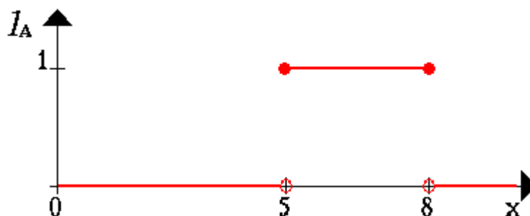
2.1. Зображення приналежності звичайної (чіткої) множини
