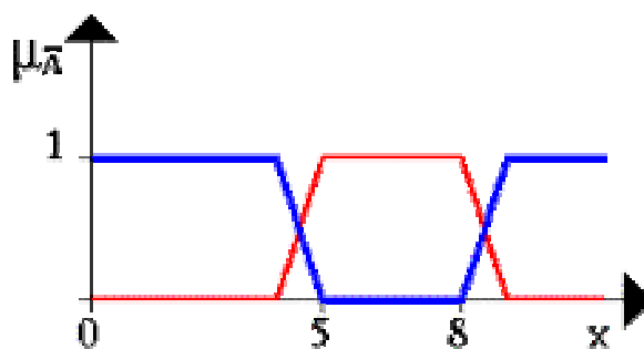
Рис. 2.11. Ілюстрація операції доповнення нечіткої множини A
