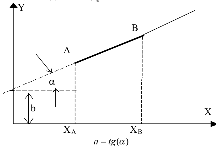
Рис. 6.1. Приклад опису відрізка AB
