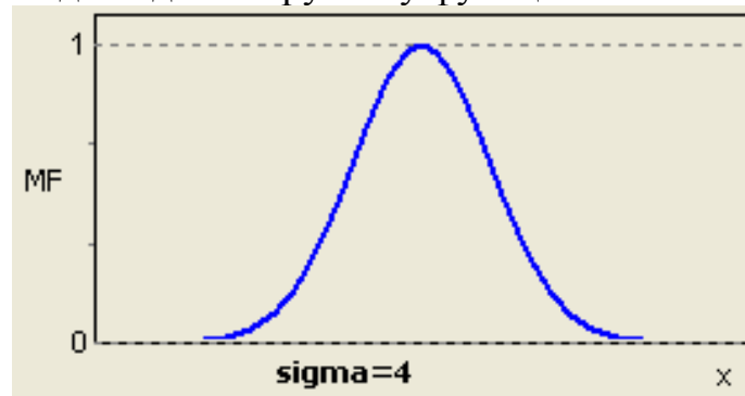
Рис. 2.6. Гауссова функція приналежності.
