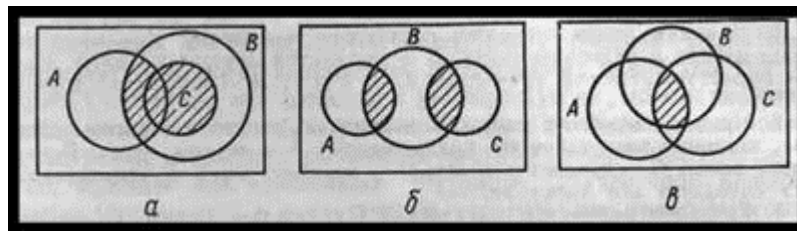
Рис.1 Круги Ейлера до завдання 12.
