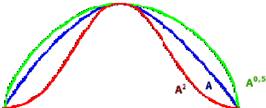
Рис. 2.13. Операції концентрації CON(A) та розмивання DIL(A)
