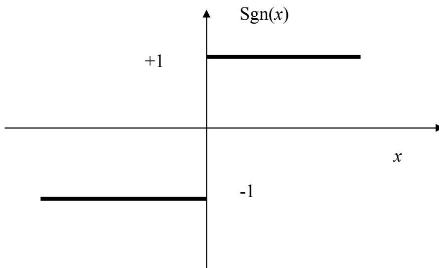
Рис. 6.3. Вигляд функції \text{sgn}(x)
