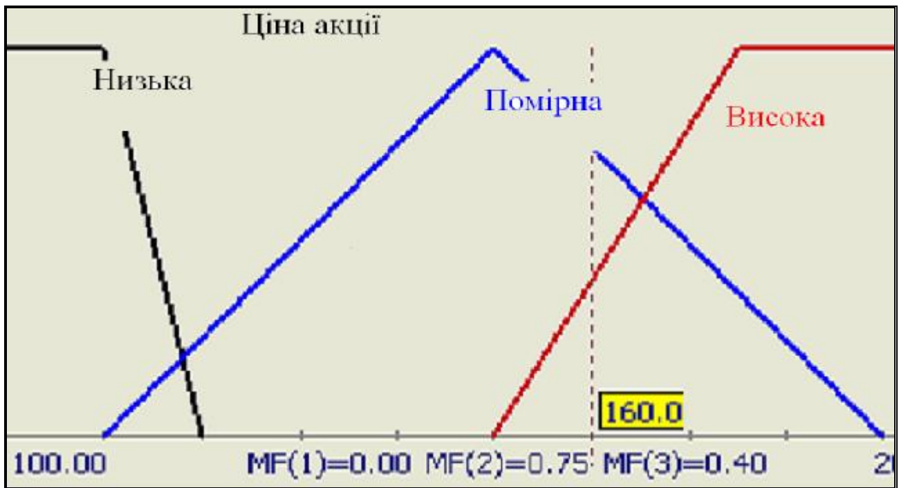
Рис. 2.7. Опис лінгвістичної змінної «Ціна акції».
